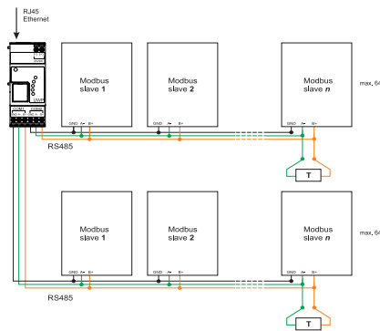
Fig. 1 Connexion Modbus RTU. COM 1 maître, COM 2 maître
