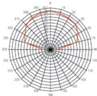
Directivité à 1kHz
