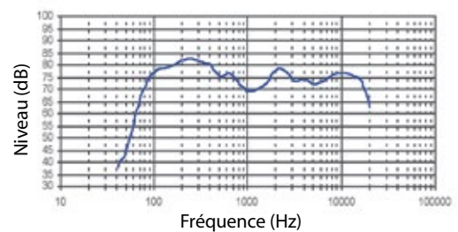
Réponse en fréquence
