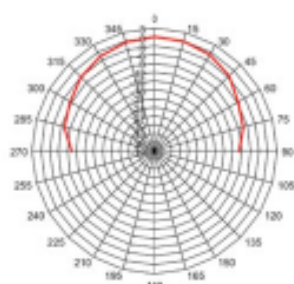
Directivité à 1kHz
