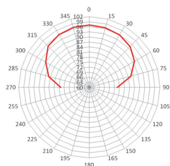
Directivité à 1kHz
